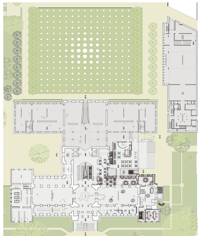
Grundriss EG
